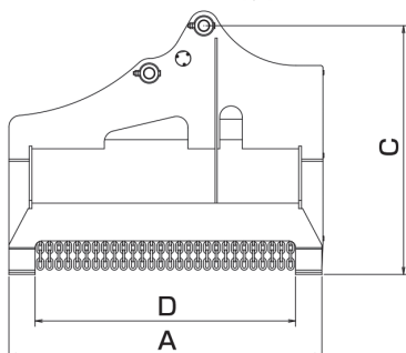
■クサカルゴン 仕様図
