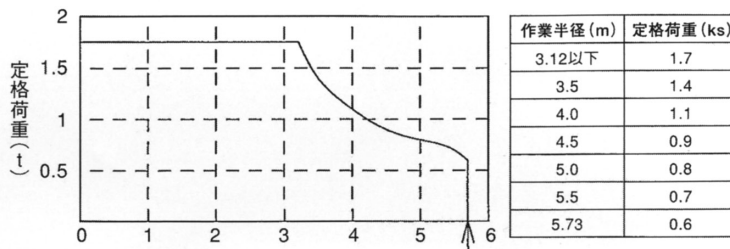
■ 定格荷重曲線 308CCR (BOX式スライドアーム・ショベルクレーン) 定格荷重表
