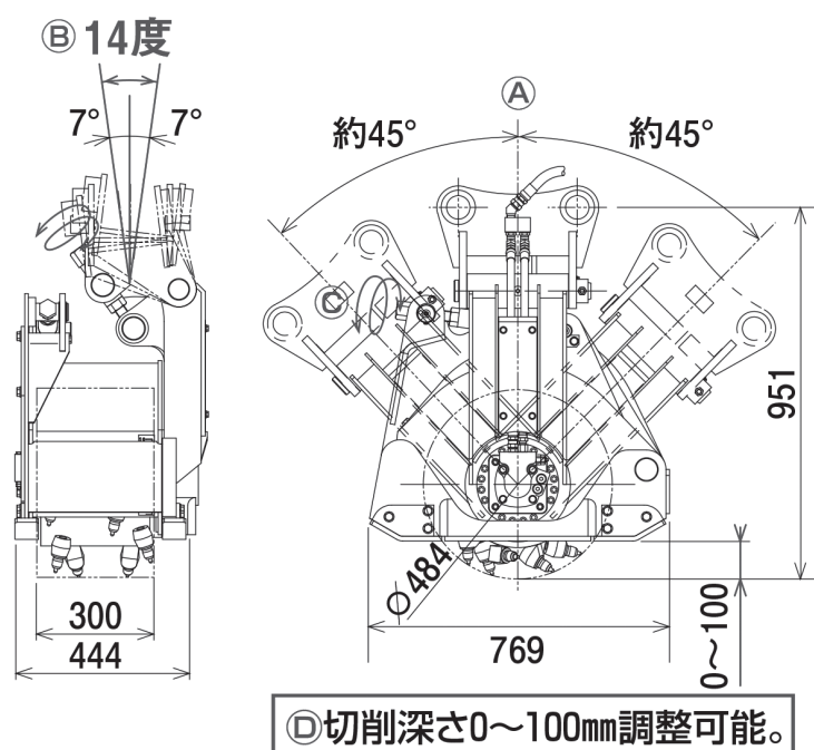
■エスカルゴン仕様図 (mm)
